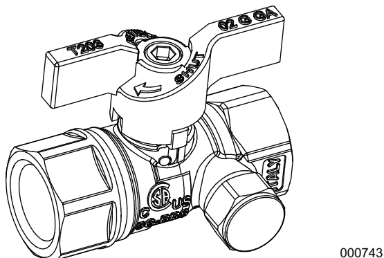
Figura 5-2. Válvula de accesorio con lumbra para manómetro
